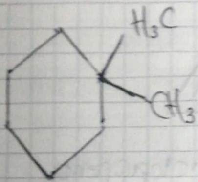
3,3-dimetil-ciclohexano
