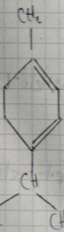
1-isopropil-4-metil-1,3-ciclohexeno
