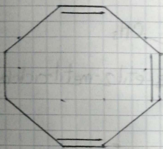
1,3,5-cicloheptatrieno
