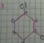
1,3-dimetilclorobenceno m-diclorobenceno
