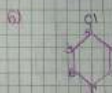
1,2,3-triclorobenceno
