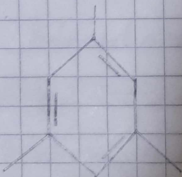
1,3,5 trimetilbenceno
