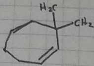
3,3 Metil ciclohepteno
