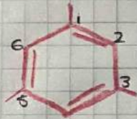
1,3,5-trimetil-benceno
