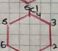
1-bromo-4-cloro-benceno
