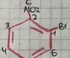
1-bromo-2-nitro-benceno (o-bromo-nitro-benceno)
