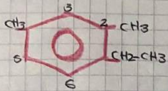
1-etil-2,4-dimetil-benceno.
