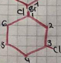
1,3-dicloro-benceno.
