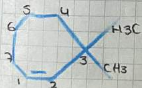
3,3 dimetilciclohepteno
