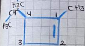
4 etil-1 metilciclobuteno
