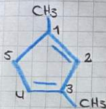
1,3 dimetil-1,3-ciclopentadieno
