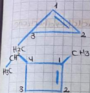
4 etil-1 metilciclobuteno
