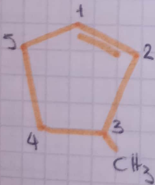
3 metil ciclopenteno.
