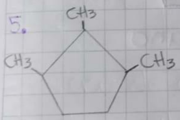
1,2,3-trimetilCiclopentano
