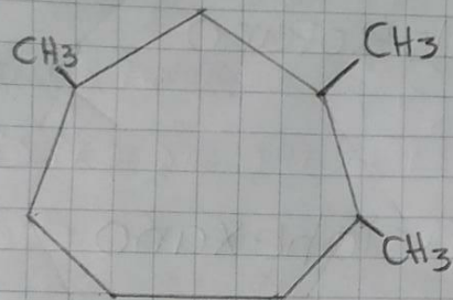
1,2,4-trimetilcicloheptano
