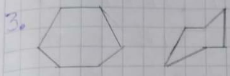
Ciclohexano
