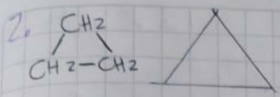
Ciclopropano
