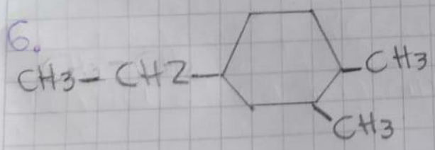
4-Etil-1,2-dimetilCiclohexano
