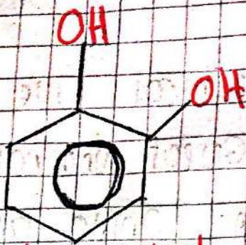
ORTOFENOL DIOL 1,2-benzenediol
