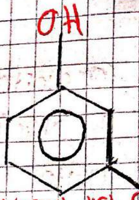
METAFENOL DIOL 1,3-benzenediol
