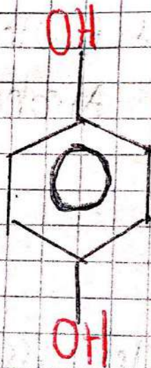
PARAFENOL DIOL 1,4-benzenediol
